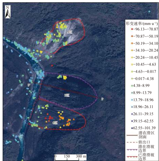
图 4 绞东滑坡形变速率图(2019 年 10 月 3 日至 2020 年 7 月 29 日, LOS 方向) Fig. 4 Deformation rate diagram of Jiadong landslide (October 3, 2019 to July 29, 2020, LOS direction) 注:影像底图为 GF-2 数据,时相为 2020 年 2 月 21 日。
