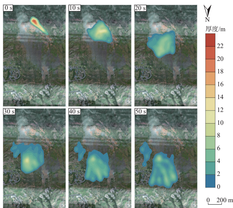
图 8 尖山营潜在滑坡致灾范围预测
