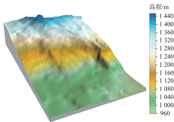
图 5 尖山营滑坡数字高程模型
