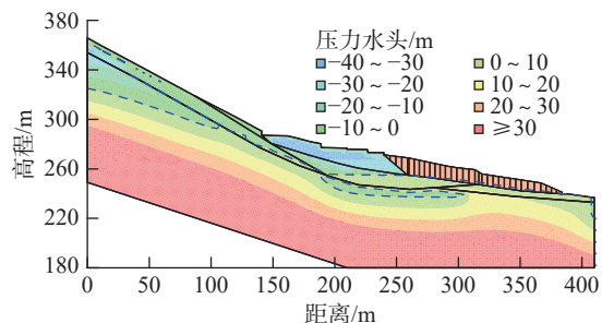
图 11 局部稳定性计算模型
