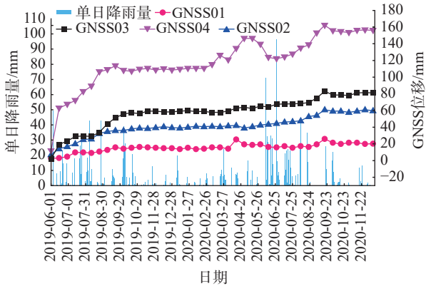
图 5 窑沟滑坡降雨量-累计位移-时间监测曲线
