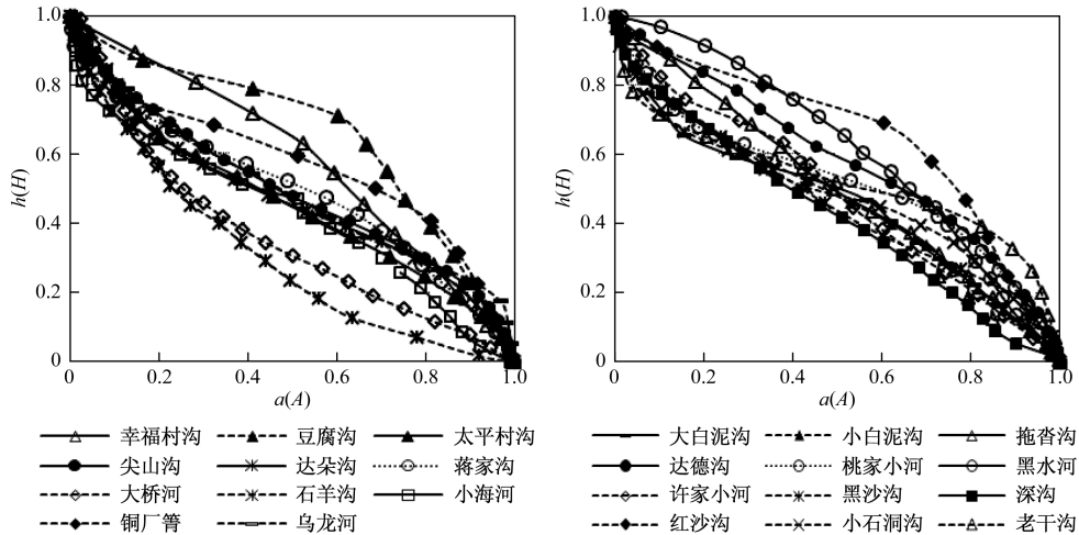
图6 小江流域泥石流沟面积~高程曲线
