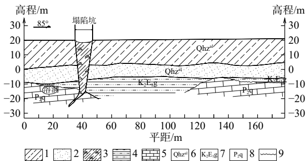
图 7 佳兆业·金城天下 3 期岩溶塌陷地质剖面图
