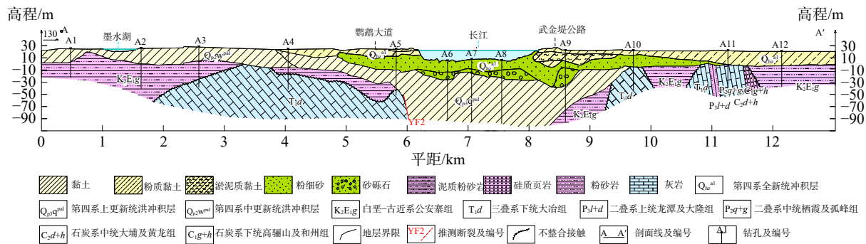
图2 研究区水文地质剖面图
