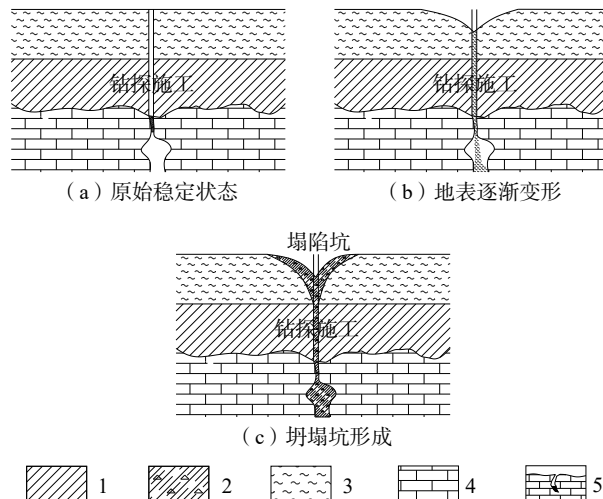
图 8 泥流型岩溶塌陷地质模型示意图
