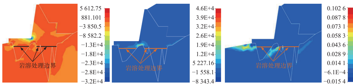
(a) 换填3 m时的挡墙大主应力(左)、小主应力(中)及体积塑性应变(右)等值线图
