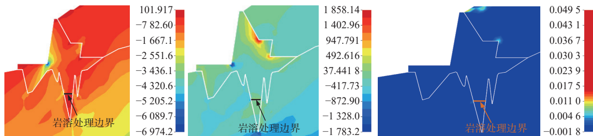
(b) 换填15 m时的挡墙大主应力(左)、小主应力(中)及体积塑性应变(右)等值线图
