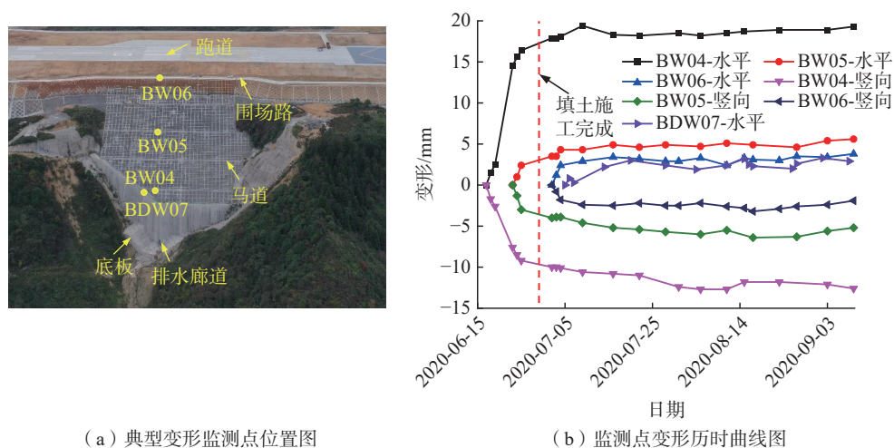
图 10 监测点位置图及其变形时程曲线
