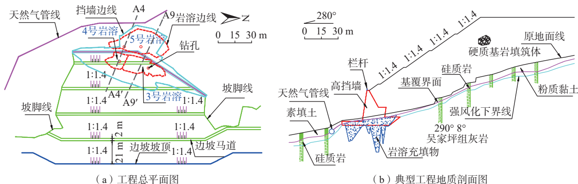
图 2 工程总平面图及典型工程地质剖面图
