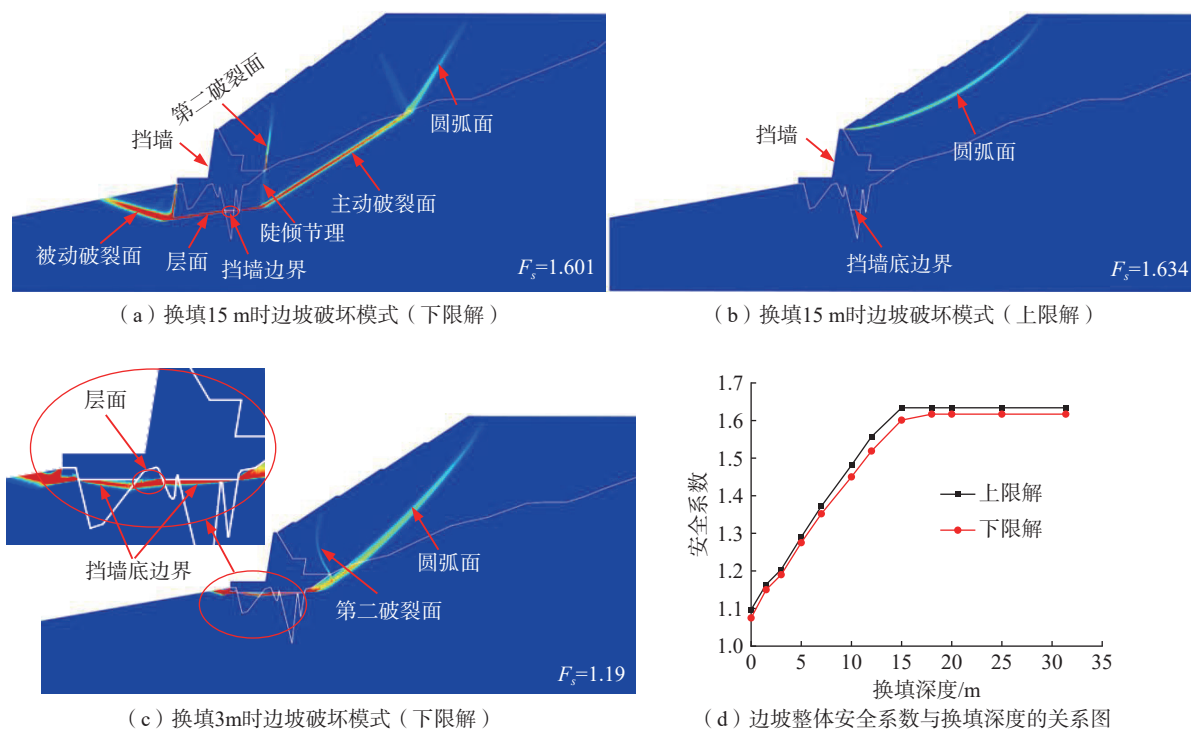
图6 不同换填深度下边坡破坏模式及整体稳定性
