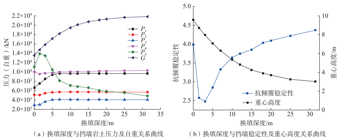
图9 换填深度与挡墙受力及挡墙稳定性关系曲线
