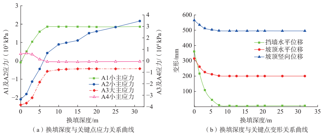
图 8 换填深度与关键点应力及变形关系曲线
