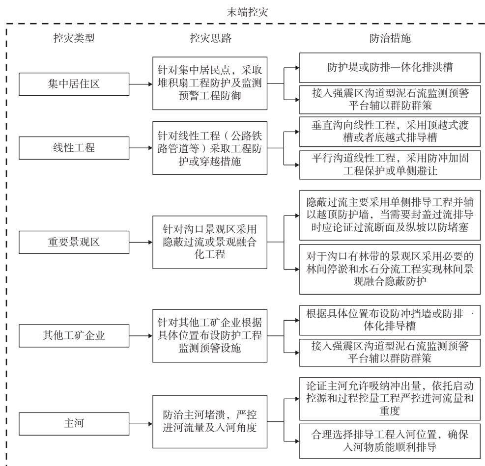
图 5 “末端控灾”关键技术体系框架图
