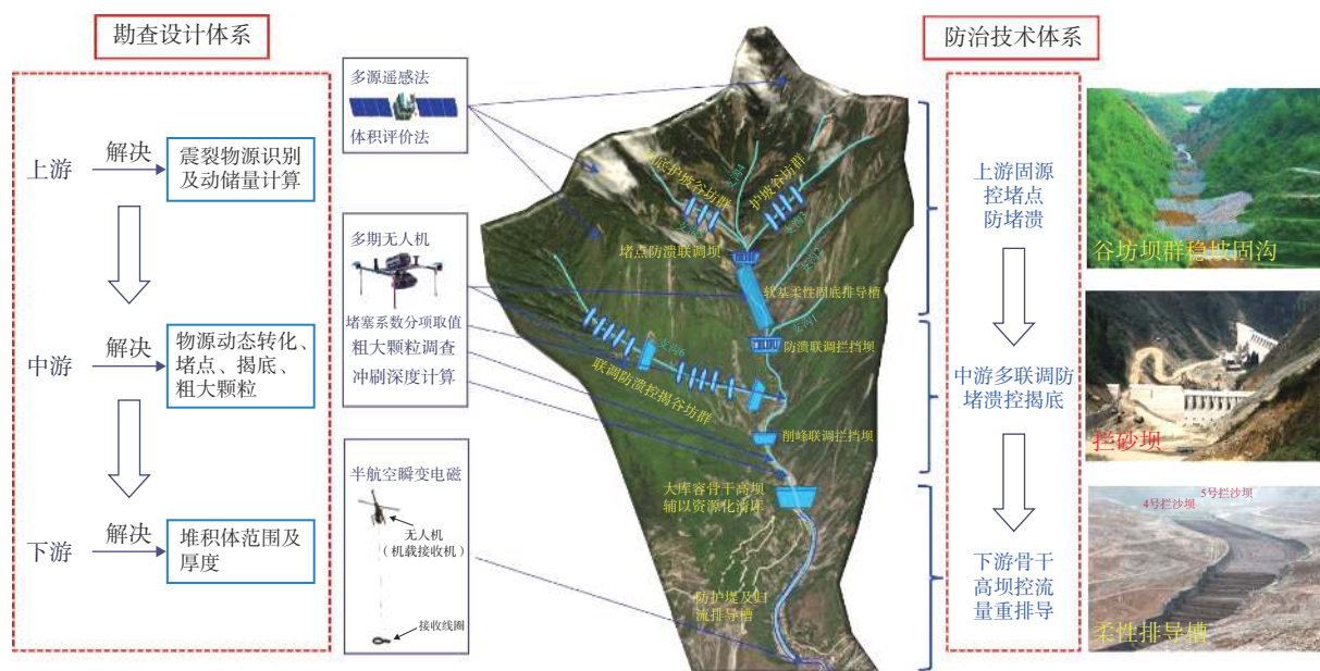
图 7 宽缓型泥石流综合防治体系示意图
