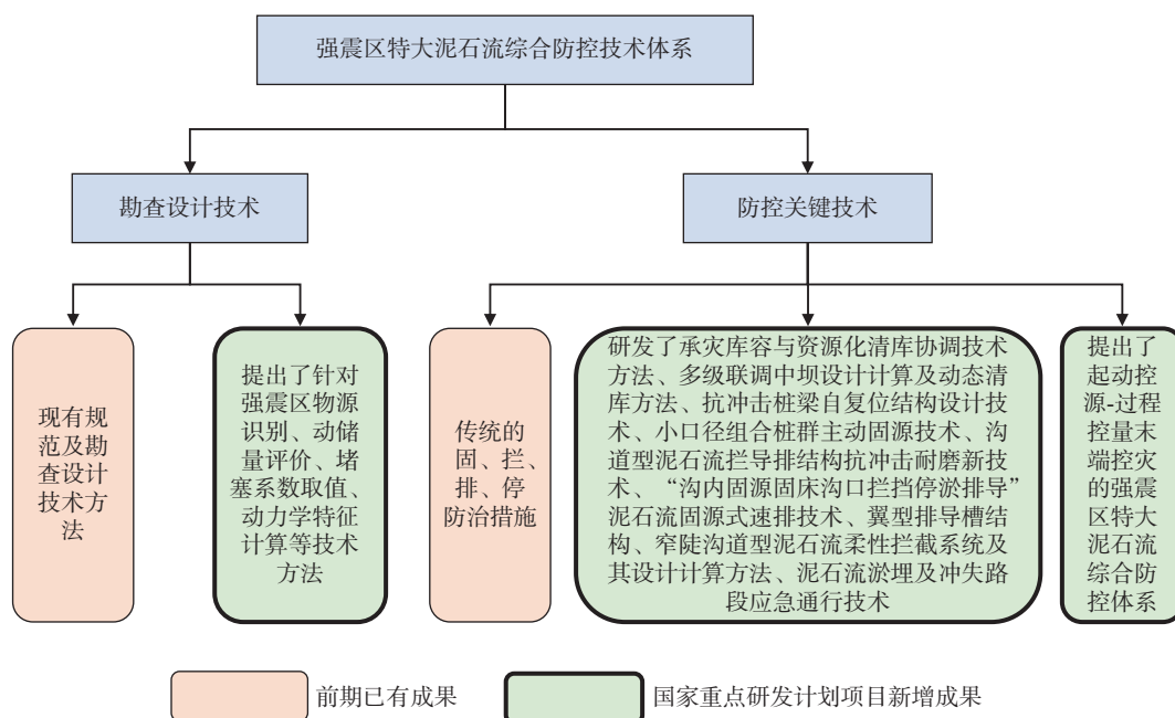
图 1 综合防控技术体系总体框架图
