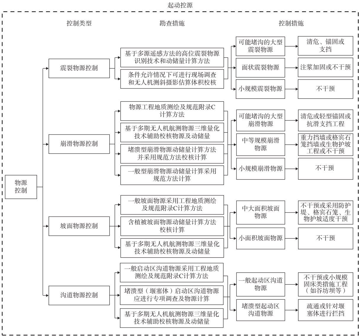
图 3 “起动控源”关键技术体系框架图
