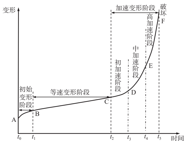
图 2 斜坡变形的三阶段演化图示 [29]
