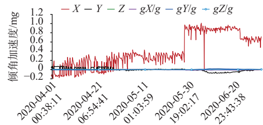
图 8 全自动 MEMS 倾角加速度累计值与时间关系曲线图 (桃树坪不稳定斜坡)
