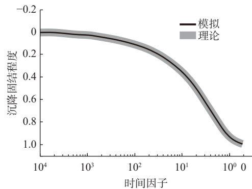
图3 固结程度和时间因子关系图(修改自文献[33])
